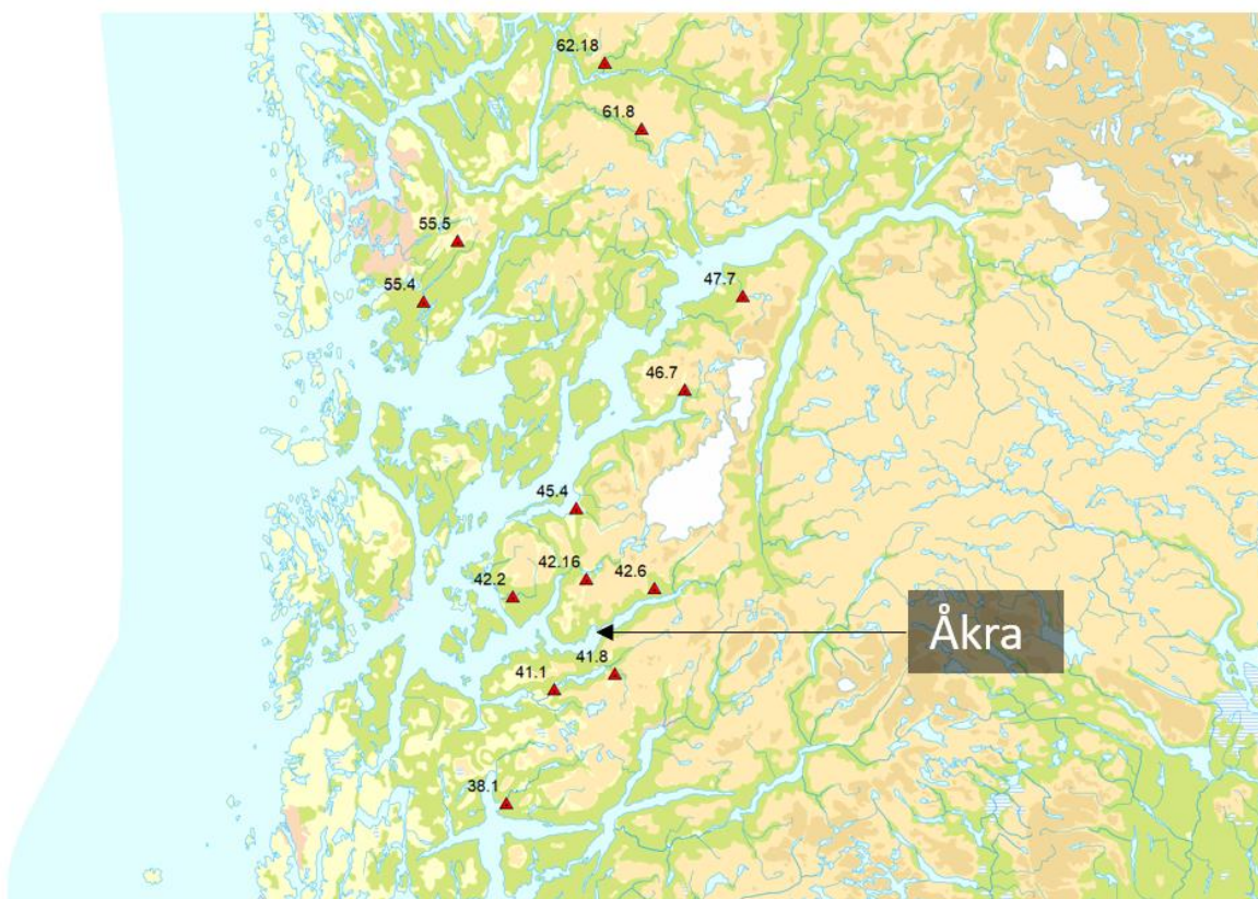
Figur 5 Vannmerker benyttet i regional flomanalyse
